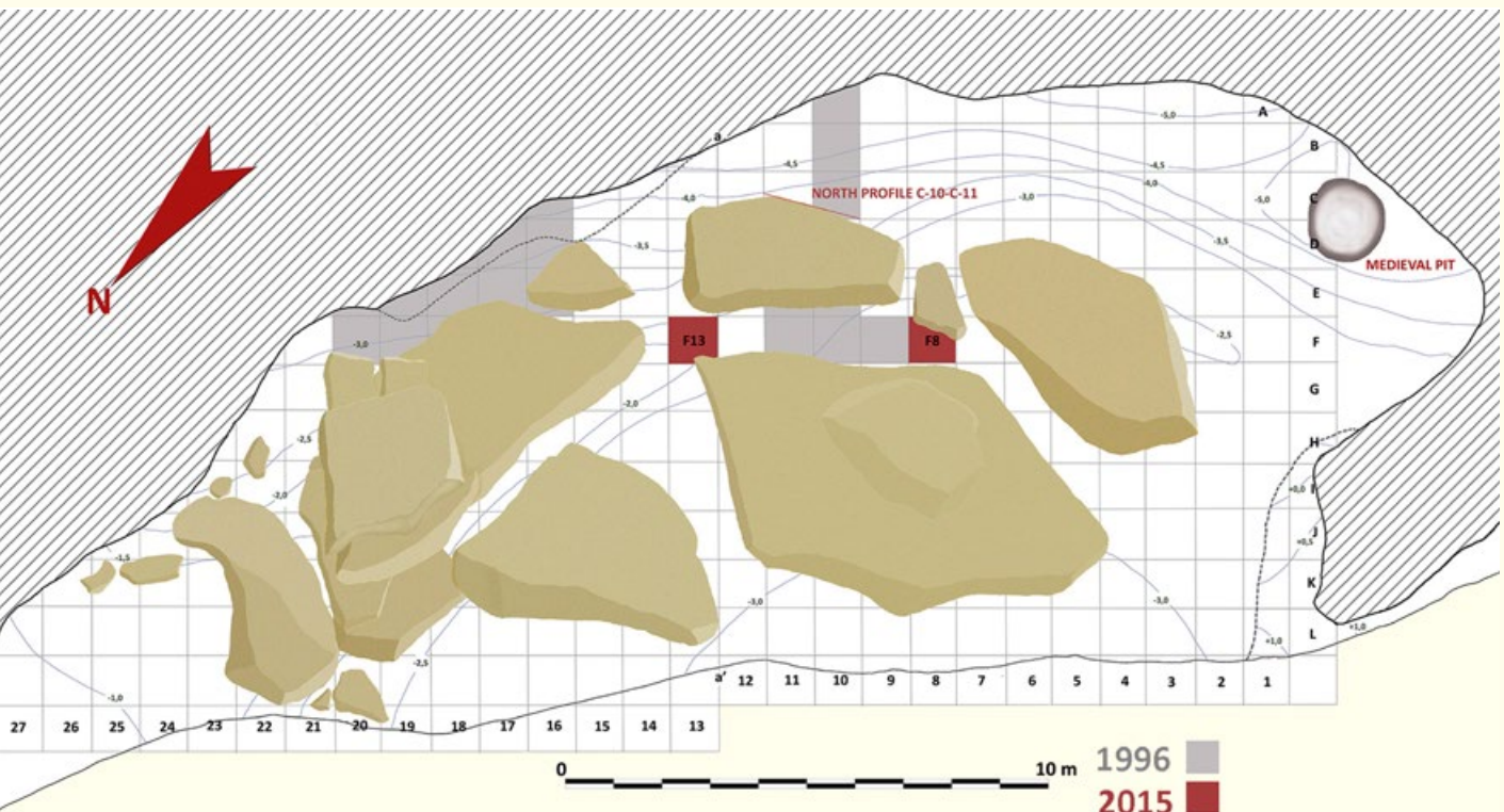
Figura 4.A: Planimetría de las excavaciones del abrigo de Peña Cabra.
