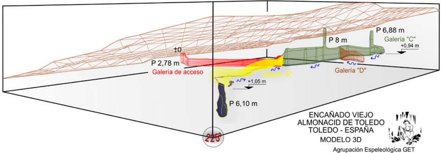
Modelo 3D del Encañado de Almonacid. Elaboración propia.
