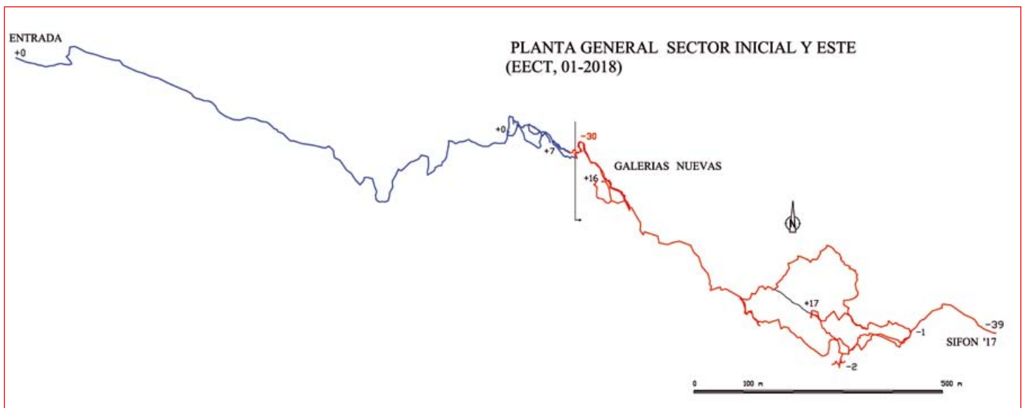
Figura 4-6. Planta general del sector Inicial y Este. En rojo las galerías descubiertas, en azul las ya conocidas. (topo EECT, 01-2018)
