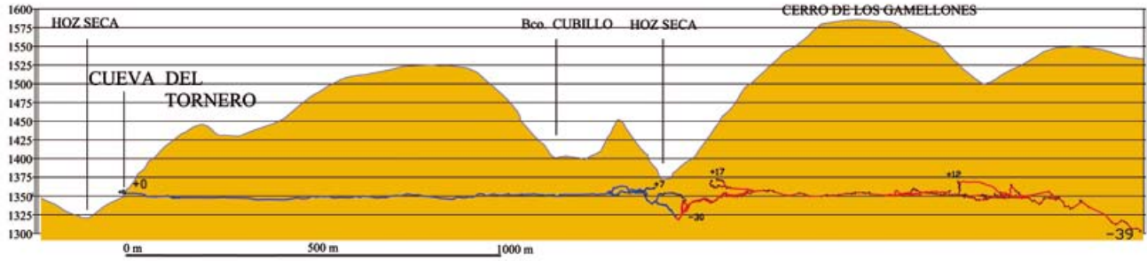
SISTEMA DE LA CUEVA DEL TORNERO. PERFIL LONGITUDINAL N° 1 (A LO LARGO DEL DESARROLLO DE LA CUEVA, poligonal azul: galerías conocidas; poligonal roja: galerías nuevas)
