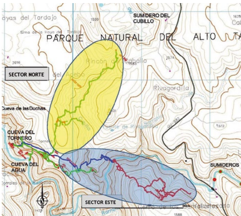
Figura 4-2. Mapa con la topografía del Tornado, en la que se señalan los grandes sectores que presenta la cueva. (en trazo verde la topo de Minas, en trazo azul y rojo la topo EECT)
