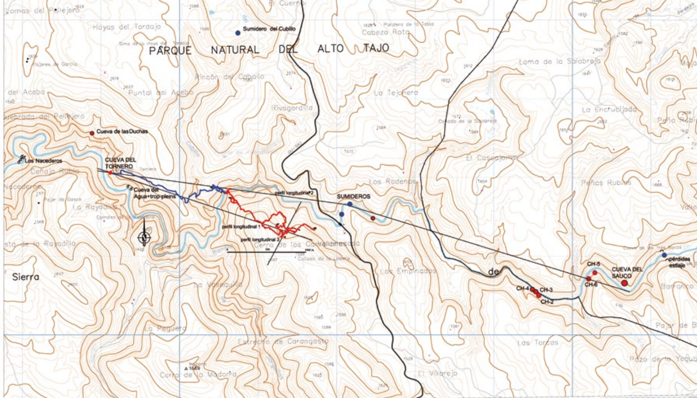
Figura 4-29. Plano general de situación, donde se muestran las surgencias, sumideros (puntos azules), cuevas exploradas a lo largo de la Hoz Seca (puntos rojos) y la planta del Tornero en su sector inicial y este (en trazo rojo las galerías nuevas, topo EECT, 01-2018). También se muestra la situación de los tres perfiles longitudinales realizados.
