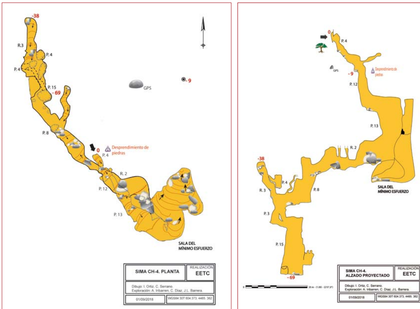
Figura 4-33. Planta de la Sima CH-4 y alzado proyectado según plano N125°E.
