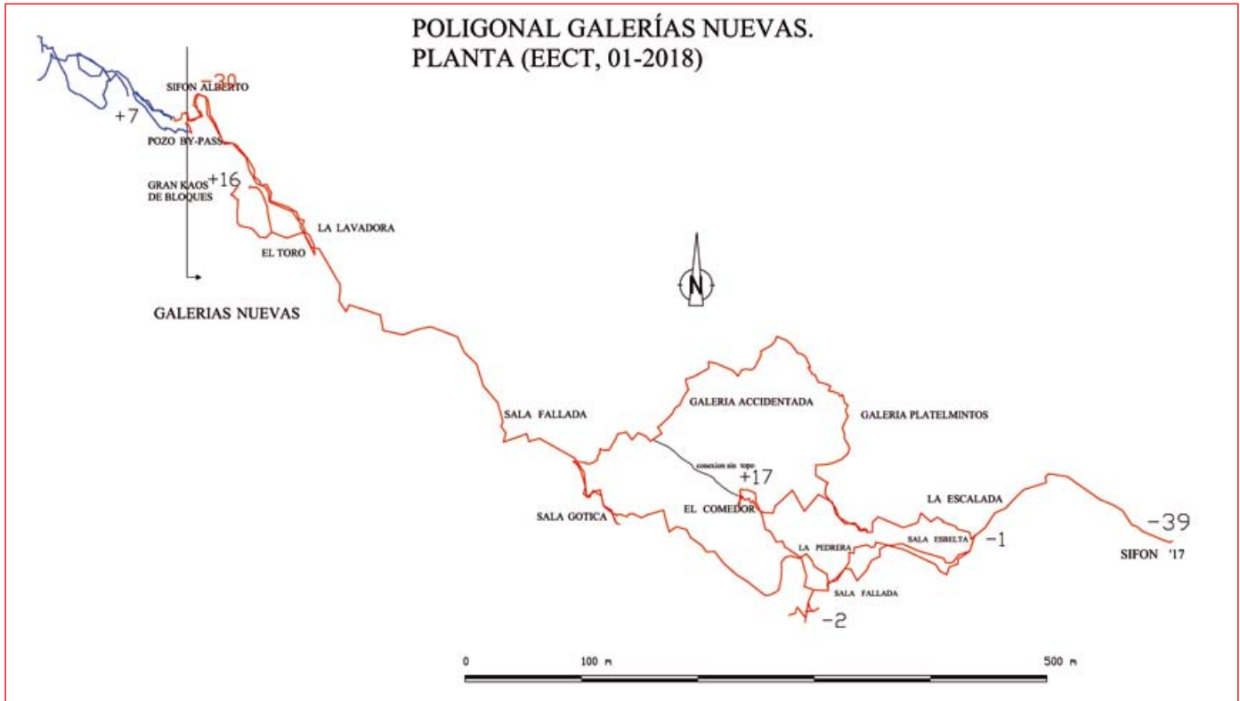
Figura 4-9. Planta topográfica con las galerías nuevas en el sector Este. (topo EECT, 01-2018)
